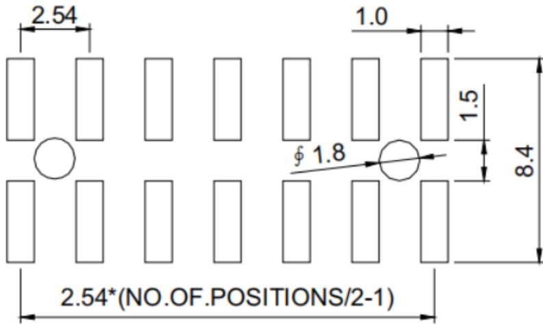
P.C.B. LAYOUT
