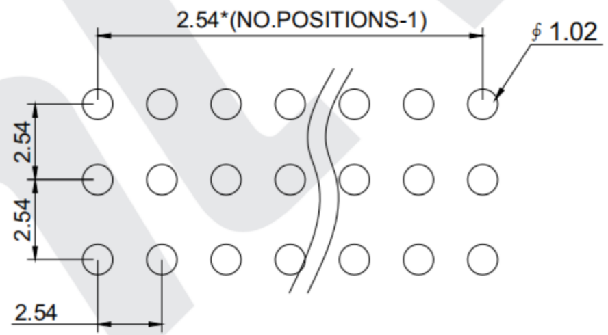
P.C.B LAYOUT
